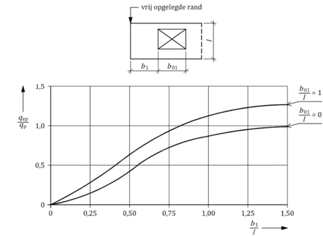
Figuur 17 — Equivalente extreme stuwdruk, q_{ep} , op driezijdig opgelegd geveldeel met breedte b_1
