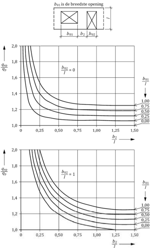
Figuur 18 — Equivalente extreme stuwdruk, q_{ep} , op penanten met een breedte b_2
