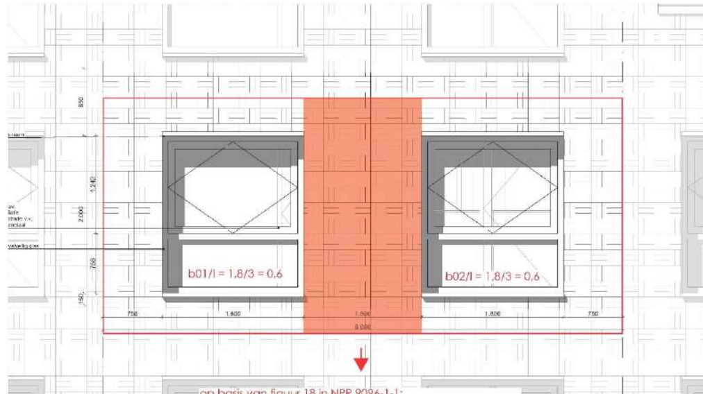
Gevelfragment 1:20 BLOK T1
