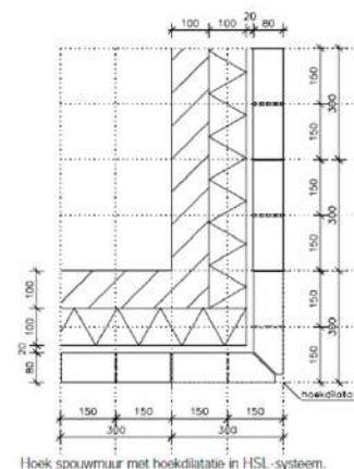
Hoek spouwmuur met hoekdilataties in HSL-systeem
